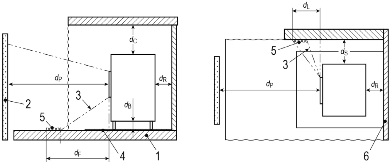
Vista laterale
